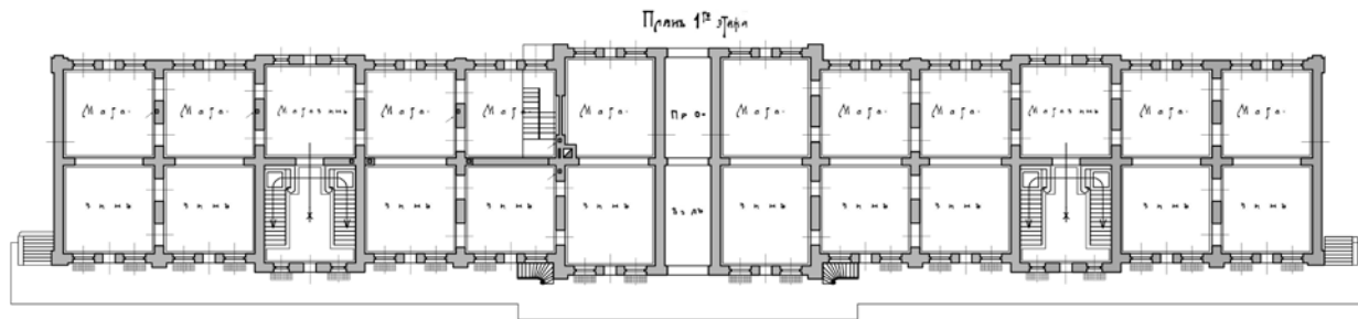
«Проект каменного 2-х этажного с подвалом Городского Торгового корпуса, предполагаемого к постройке в городе Ново-Николаевске Томской губернии по Николаевскому проспекту». Архитектор Крячков А.Д. 1910 г. «The design of the two-storied stone City Trade Building with the basement planned to be build on Nikolaevsky Prospect in Novonikolaevsk of Tomsk Province». Designed by Andrey Kryachkov, 1910.
